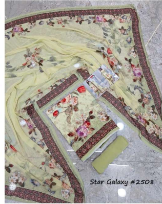
Star Galaxy #2508
